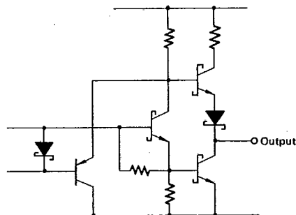
Fig. 5 - MB 7124 OUTPUT
